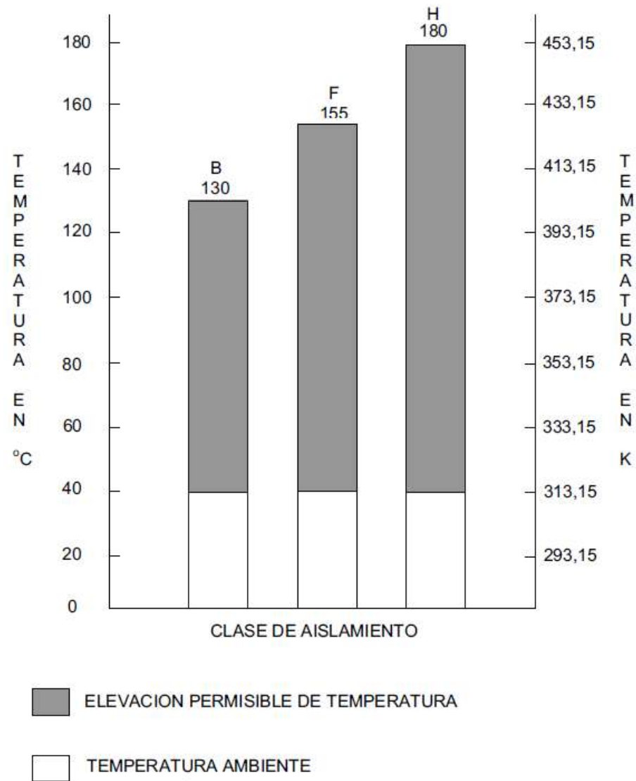
Figura 1 Temperatura para las distintas clases de aislamientos.
