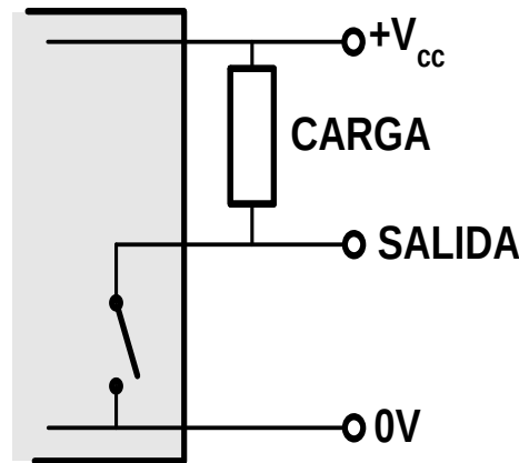
NPN
